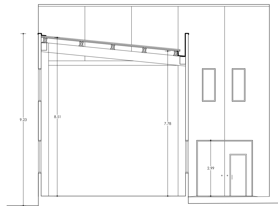
SECCIÓN A
