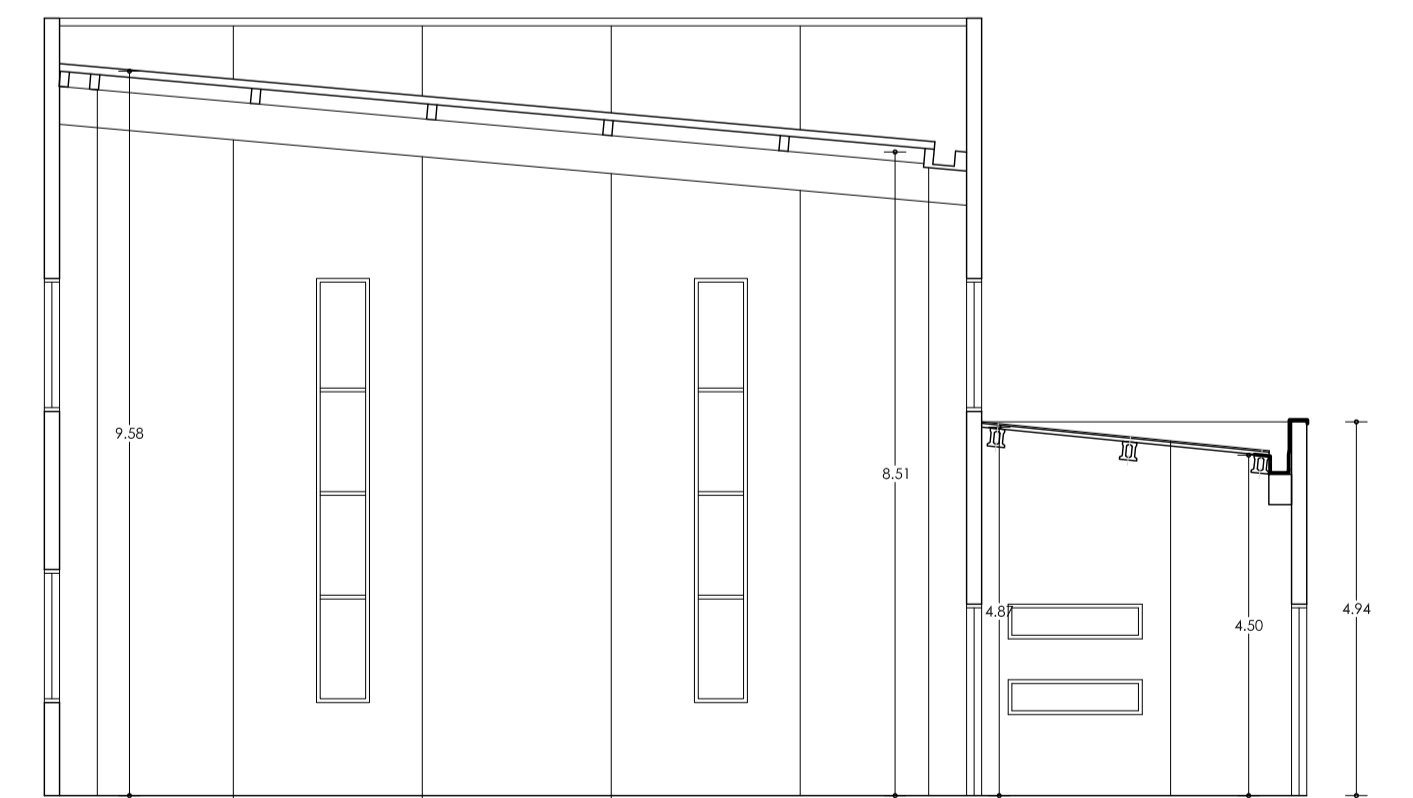
SECCIÓN B
